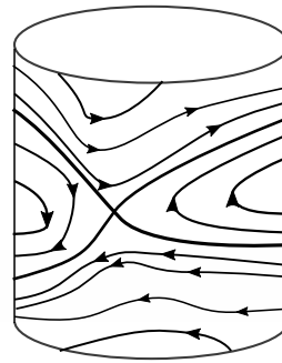
FIGURE 1 – Les courbes de niveau d'un hamiltonien sur \mathbb{T} \times \mathbb{R}
