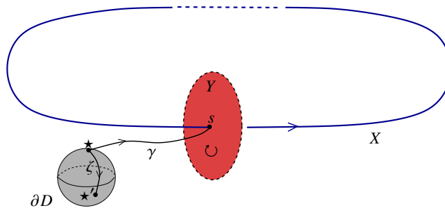
FIGURE 5.3.1. The manifold M = (S^1 \times S^{n-1}) \setminus \text{Int}(D) .
